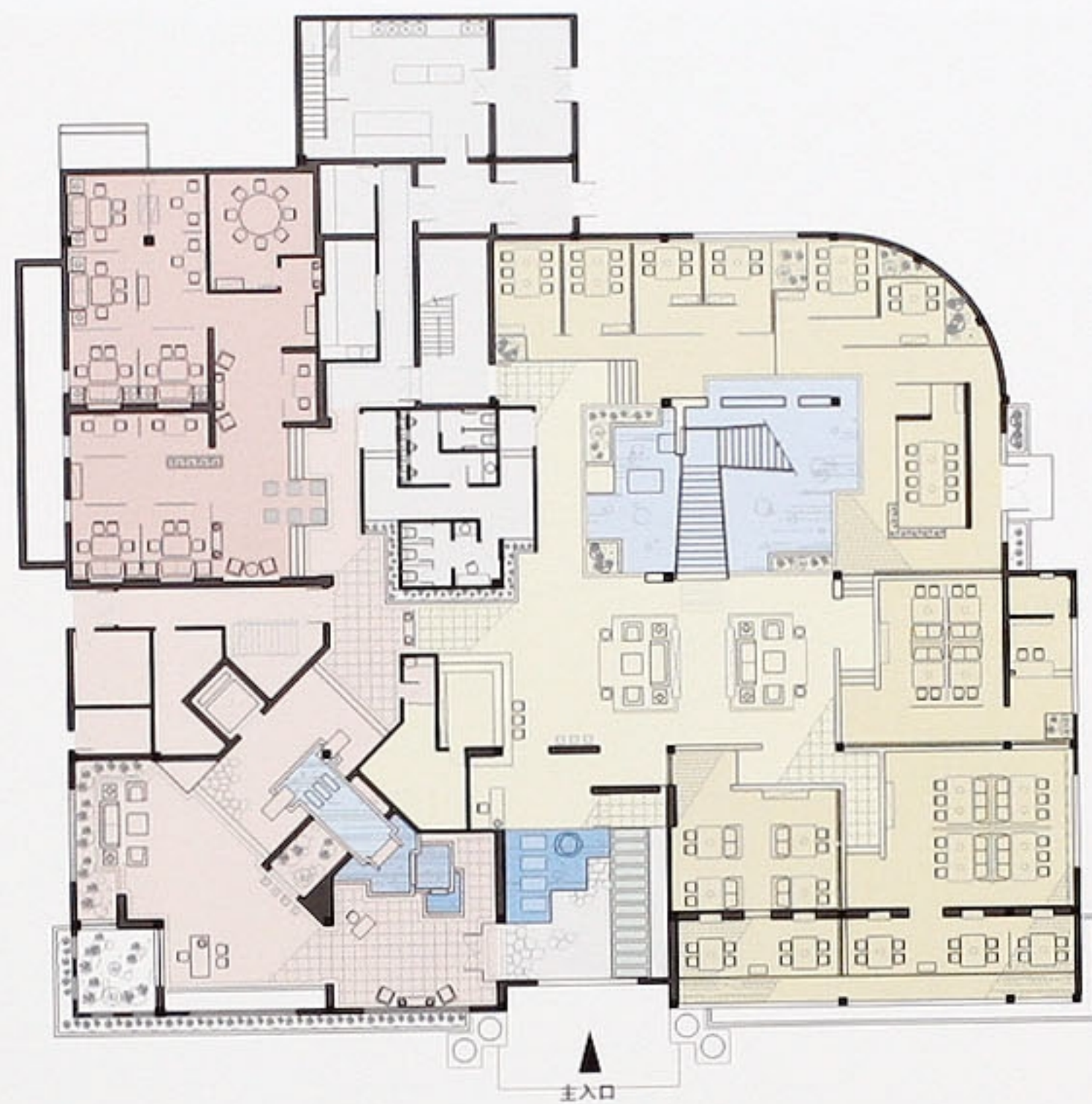
一层平面图
